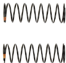
AS91958 13mm リヤスプリング 【オレンジ/2.5lb/in・L61・9.0t・1.2d】
