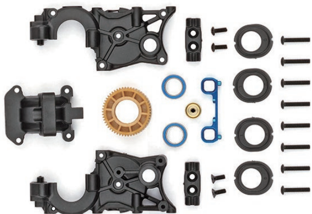
AS71220 3ギヤボックスコンバージョン【B7】
